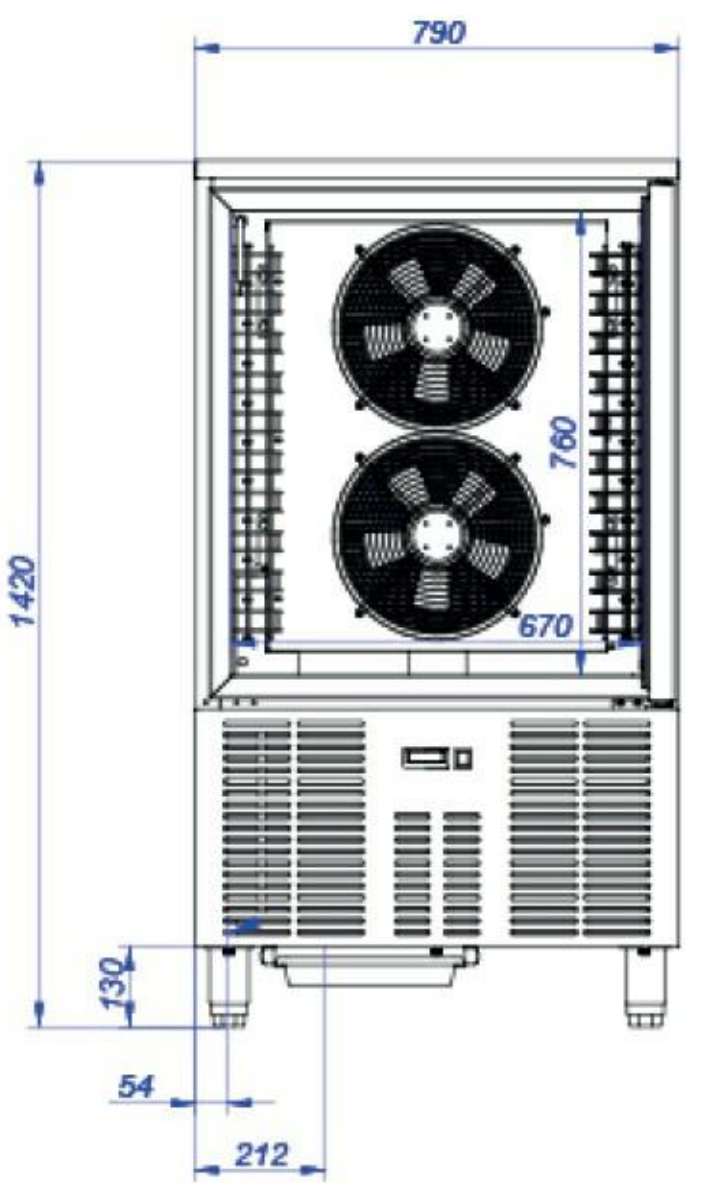
SP1050BC Dimensions
